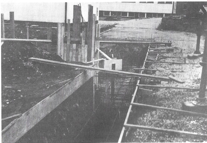
Armatura - bednění - základy DPS. Foto: Ing. Vít Kratina
